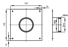
1. Króciec Pomiarowy
